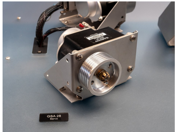
Foto real (close-up): servo Garmin GSA 28, usado pelo piloto automático GFC 500. Foto: Matti Blume – Wikimedia Commons, licença CC BY-SA 4.0.
